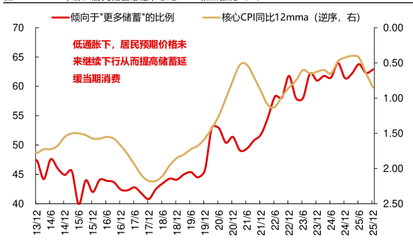
图 17：2025 年前，居民储蓄意愿和核心 CPI 相互强化（%）
